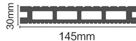
145*30mm双面方孔地板
