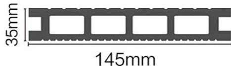
145*35mm双面方孔地板
